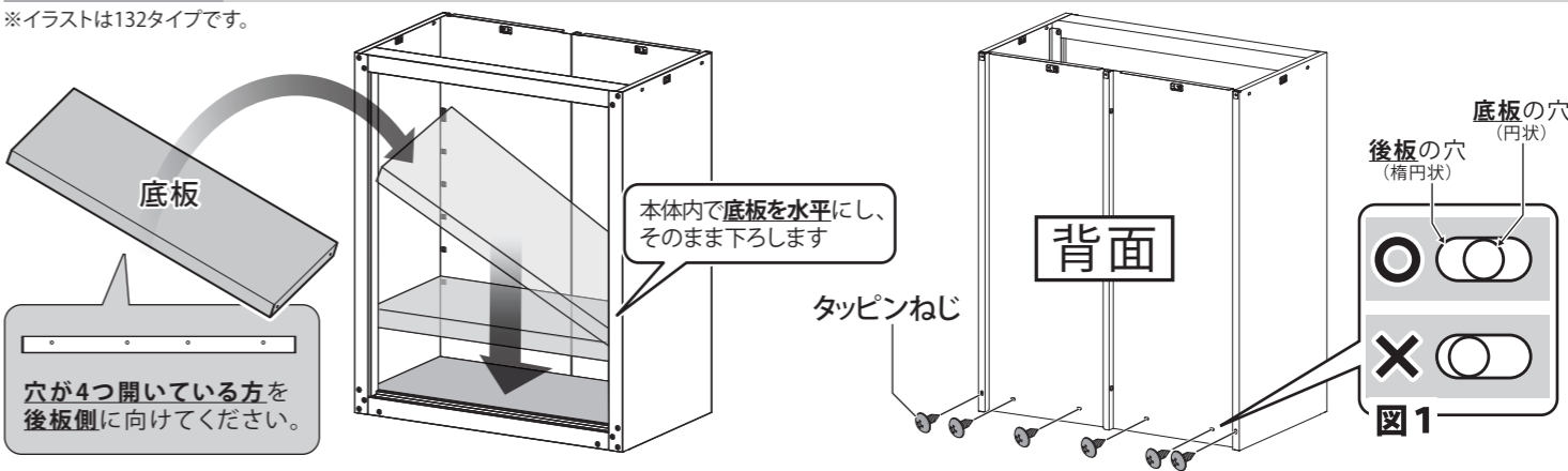
底板
