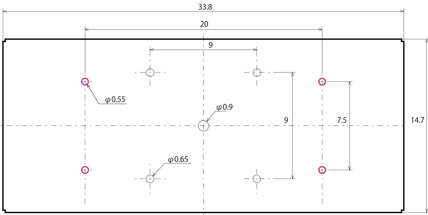
底板 (単位:cm)
