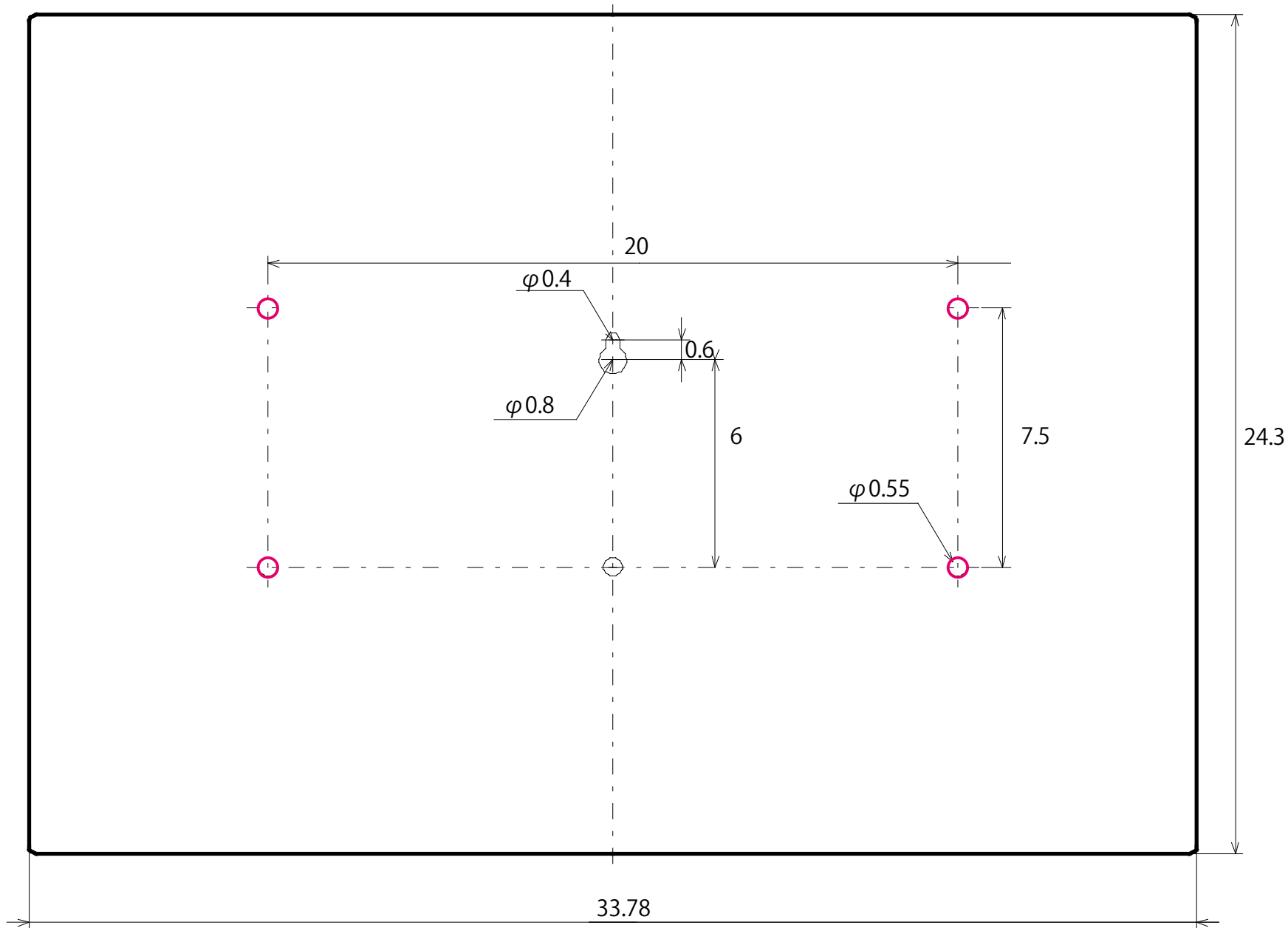
後板 (単位:cm)
